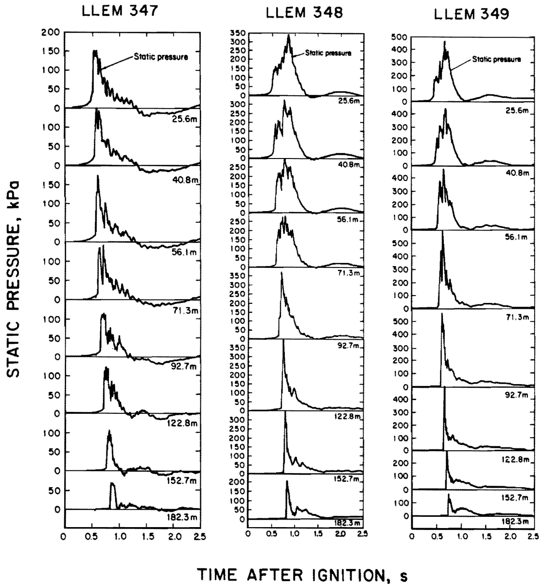
Fig. 8. Pressure wave diagrams for three explosions: LLEM test 347 ( \text{CH}_4 gas zone only), LLEM test 348 (gas plus 100 \text{ g/m}^3 coal), LLEM test 349 (gas plus 200 \text{ g/m}^3 coal).
